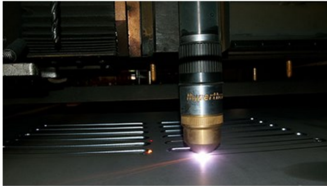
Découpe plasma 8 m*2 m avec têtes de perçage
